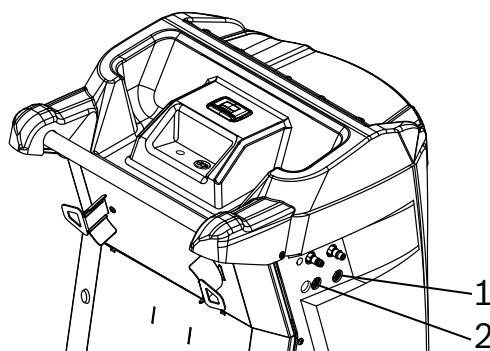
Fig. 11: Raccordement des tuyaux de service (HP et LP)
