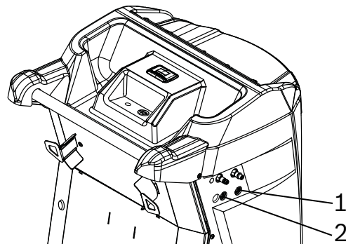
Fig. 11: Conexión de los tubos de servicio (HP y LP)
