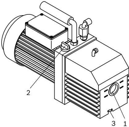
Şek. 22: Vakum pompası
