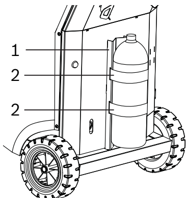
Abb. 17: Einbau des N2H2- oder N2-Tanks
