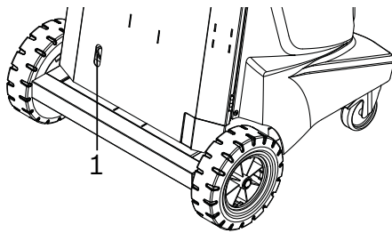
Fig. 13: Contrôle du niveau d'huile de la pompe à vide
