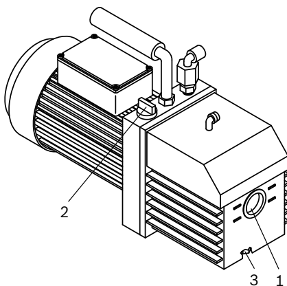
Fig. 22: Pompa del vuoto
